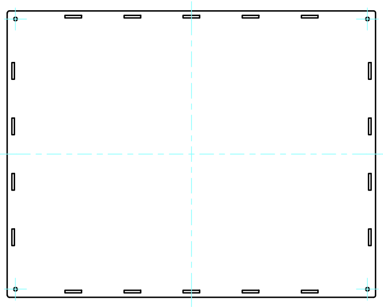
下カバー裏面 / Bottom cover Backside
