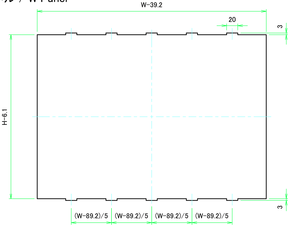
Wパネル1表面 / W Panel 1 Frontside
