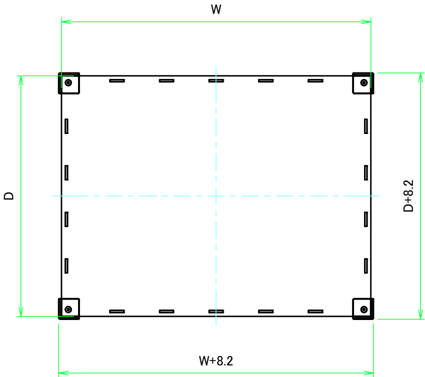
上カバー / Top cover
