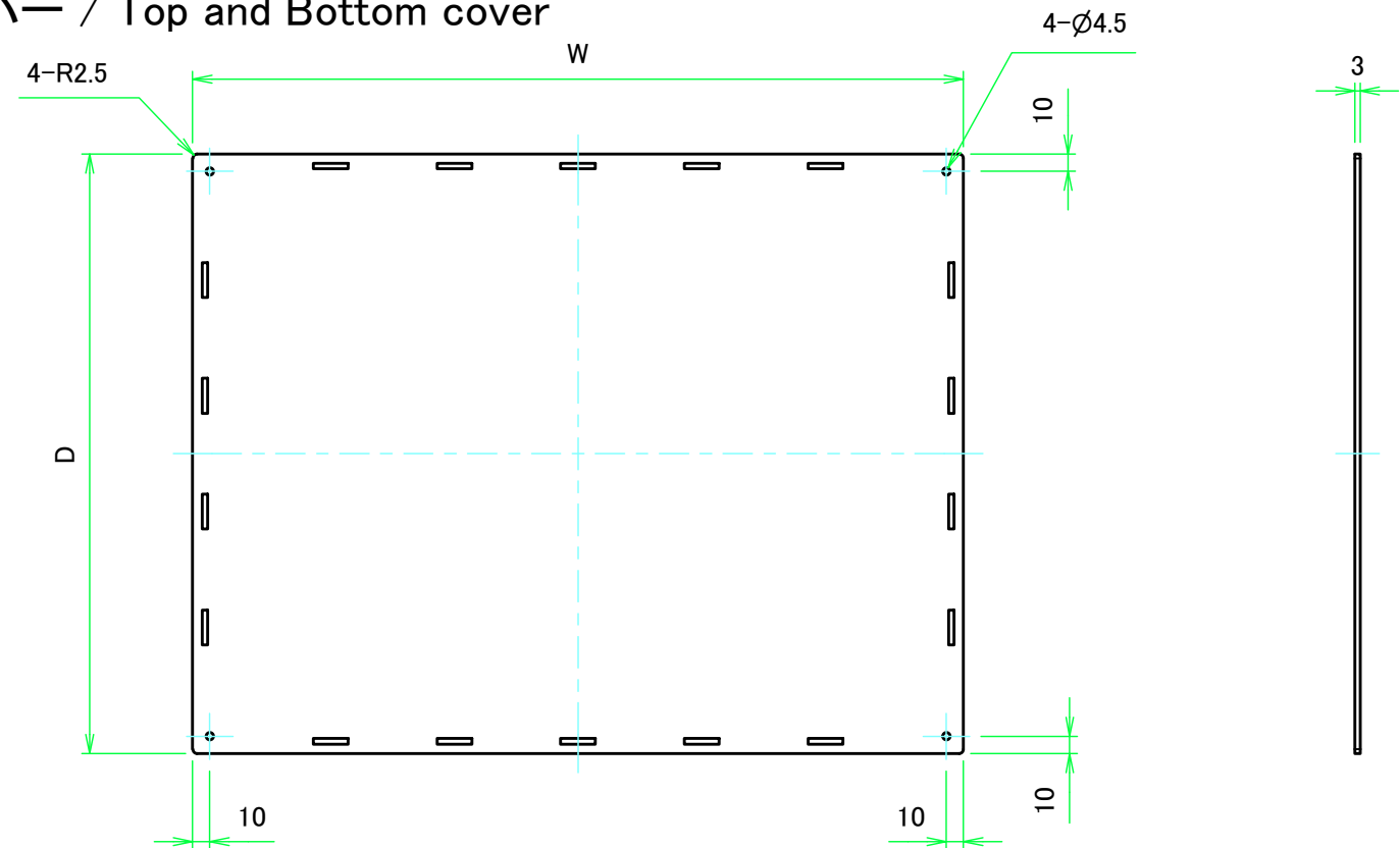
上カバー表面 / Top cover Frontside
