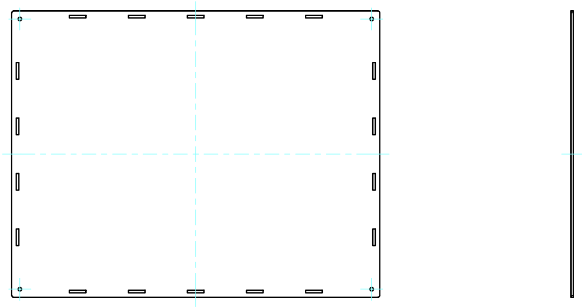
下カバー表面 / Bottom cover Frontside
