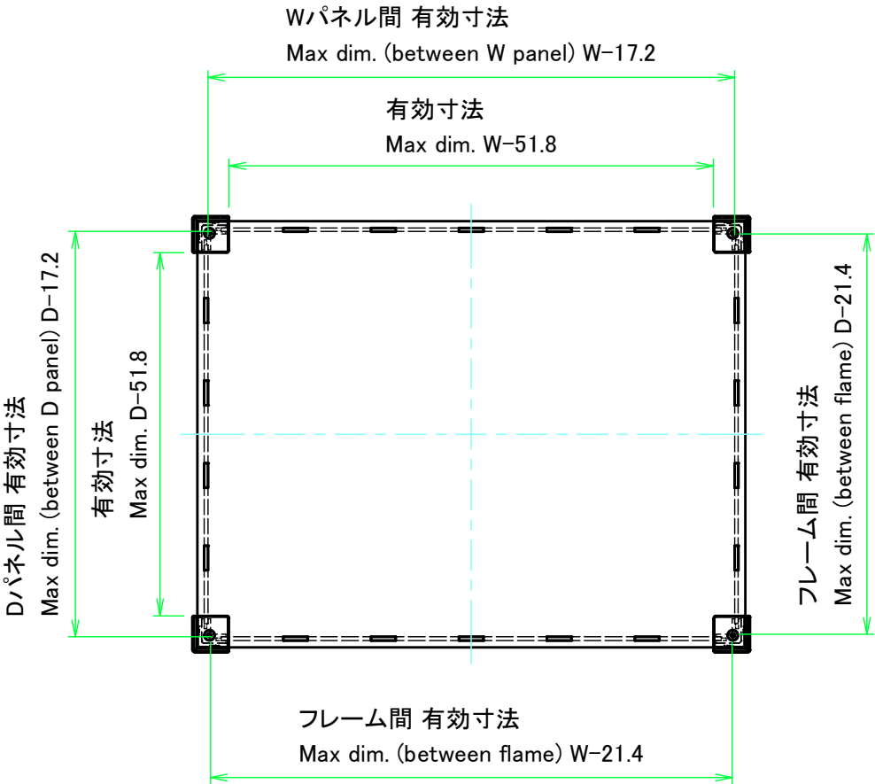
下カバー / Bottom cover
